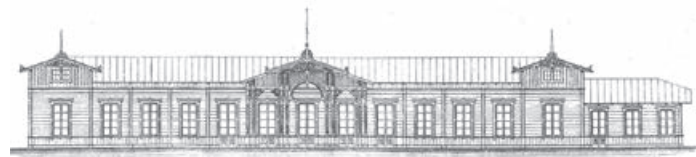
Projekt fasady drewnianego dworca D.Ż.I.D. wybudowanego w 1885 r.
