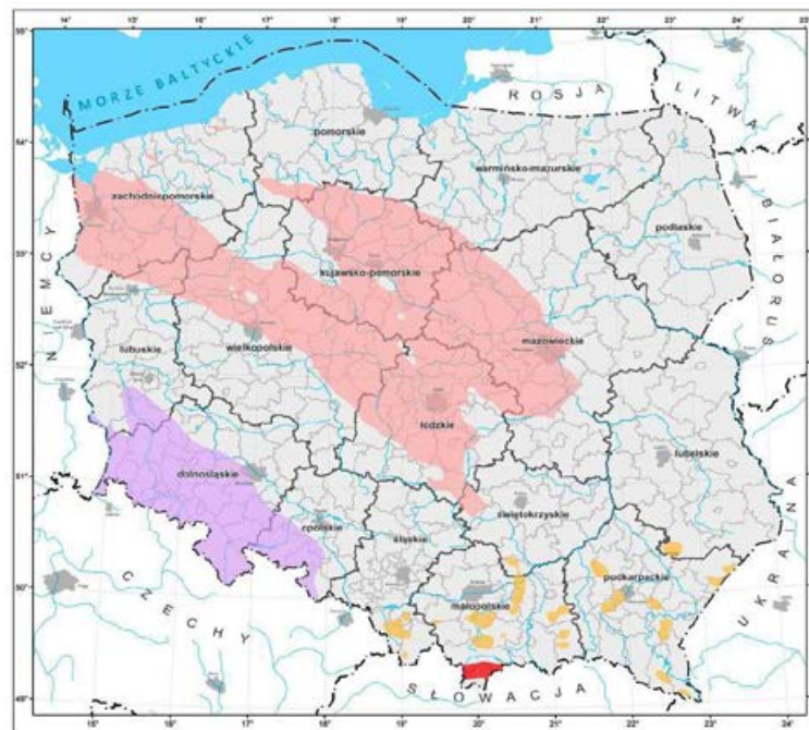
MAPA OBSZARÓW PERSPEKTYWICZNYCH DLA POSZUKIWANIA I UJMOWANIA WÓD TERMALNYCH
